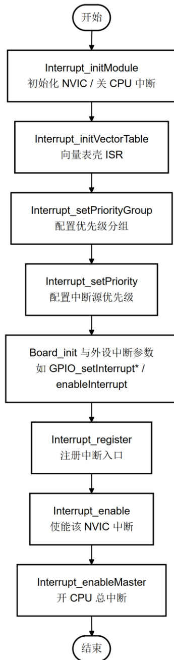
图 3 中断初始化流程
