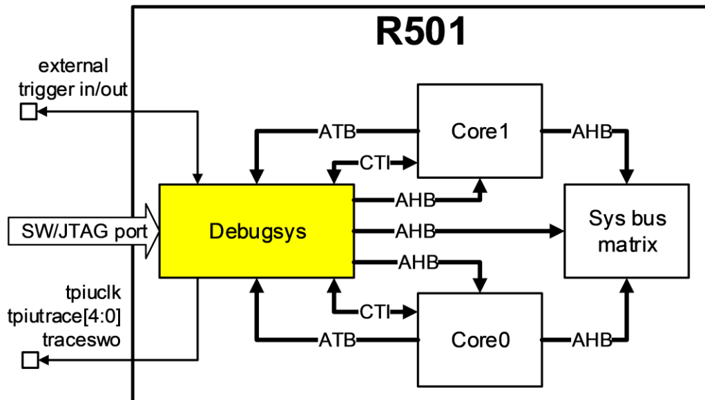
图 5 调试系统的典型集成
