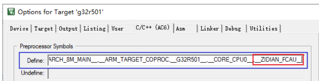
图 2 在 keil 配置界面中添加 ZIDIANFCAU 宏定义
