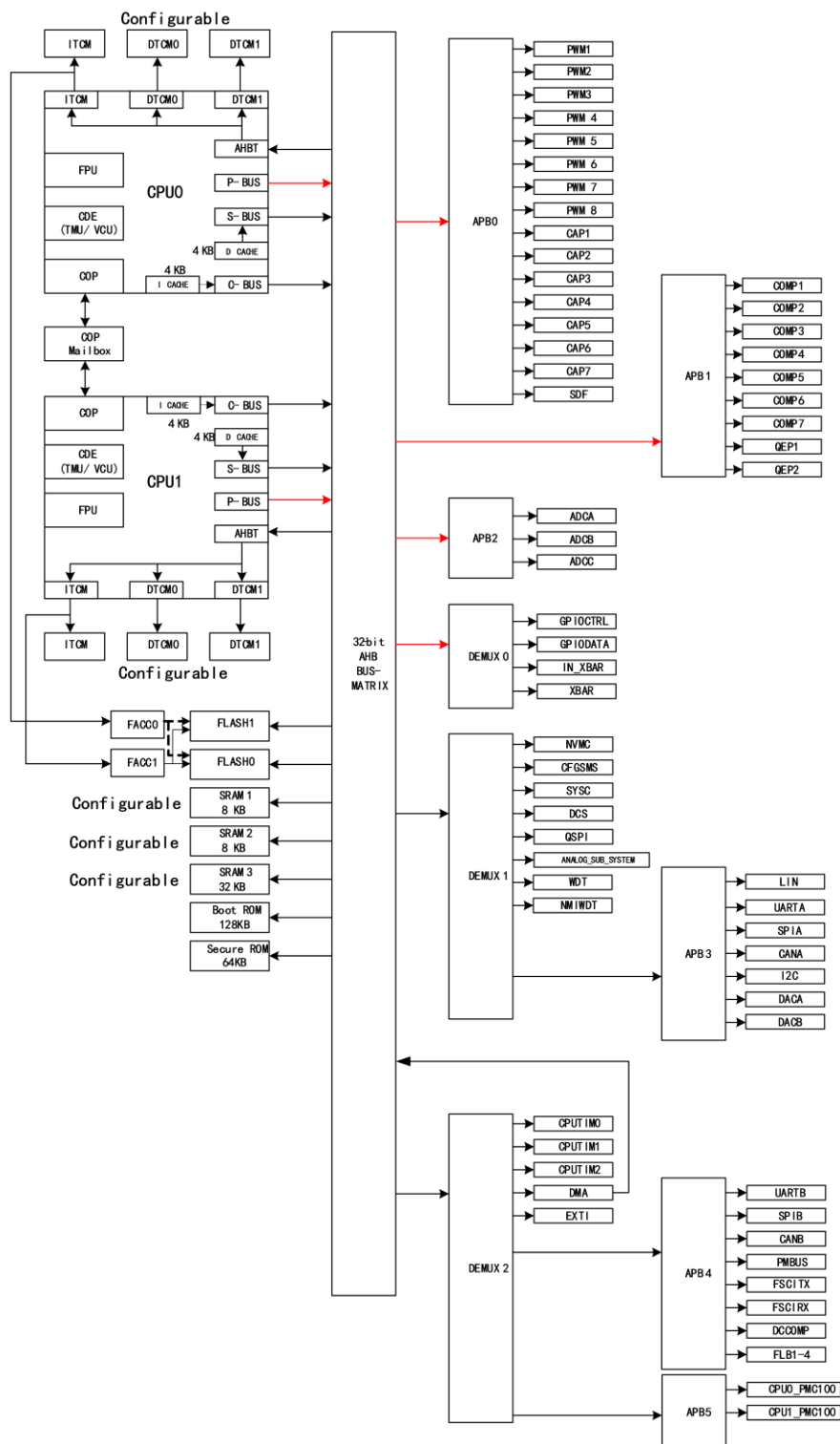
图 1 R501 SoC 架构
