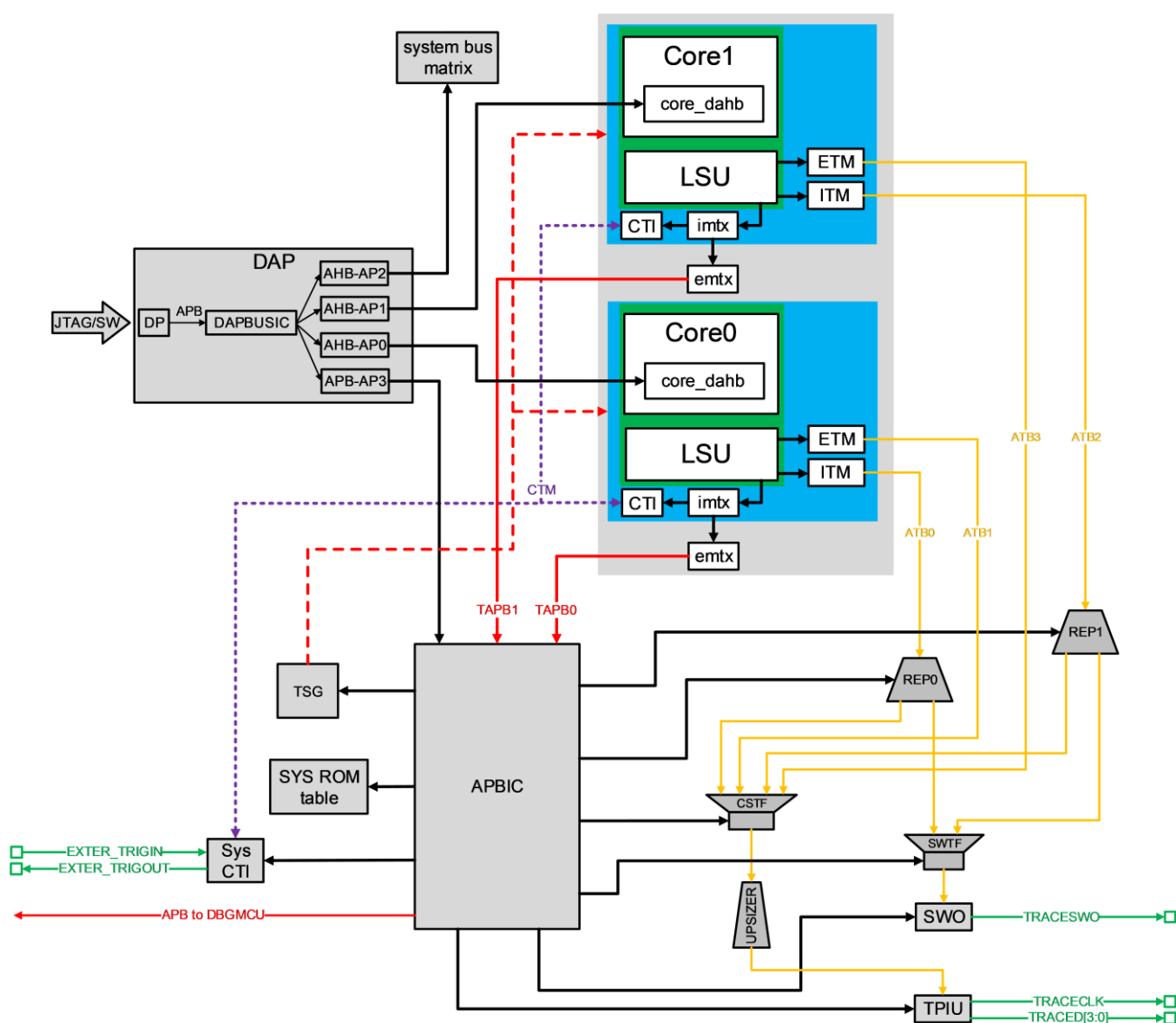
图 4 结构框图
